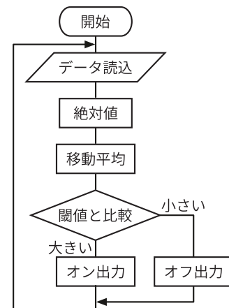
図4. オンオフ制御のフローチャート
