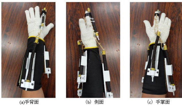
図5 作成した空気圧グローブ
